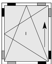
Hebe-Drehkippflügel
